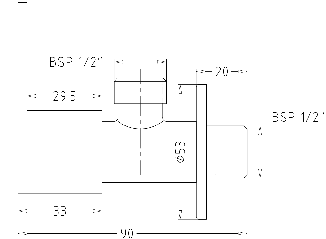
ASPIRO:F570043 ANGULAR STOPCOCK WITH FLANGE
