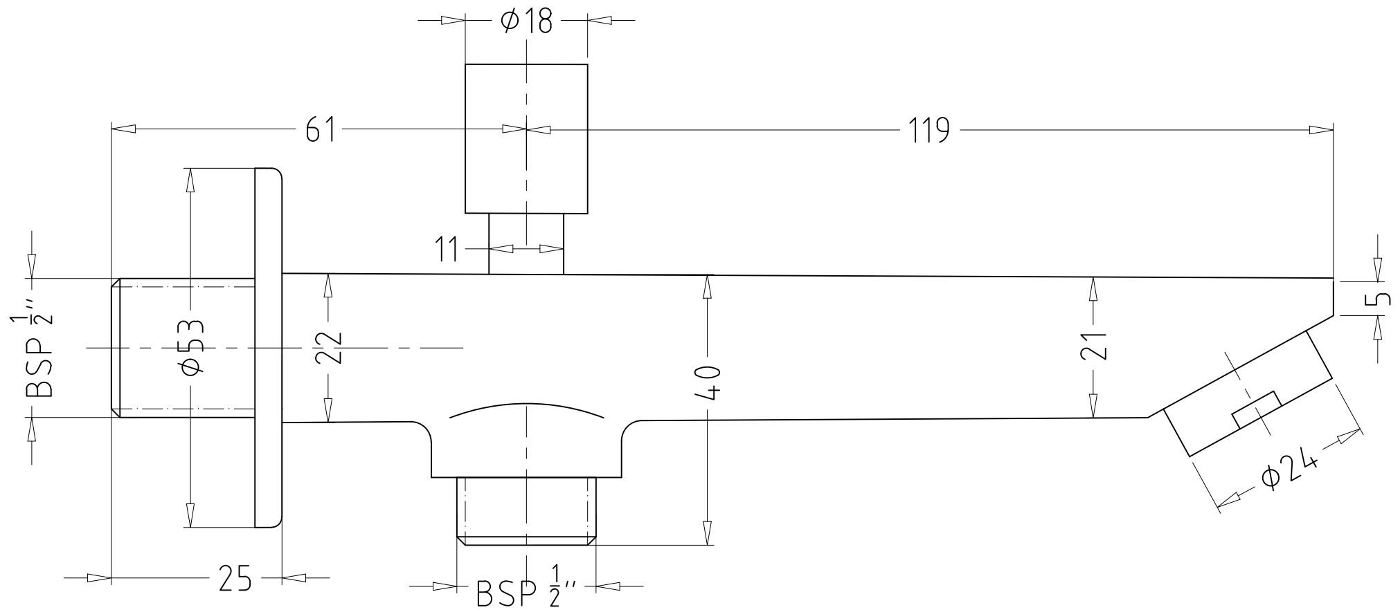
ASPIRO:F570010 BATH TUB SPOUT WITH TIPTONE
