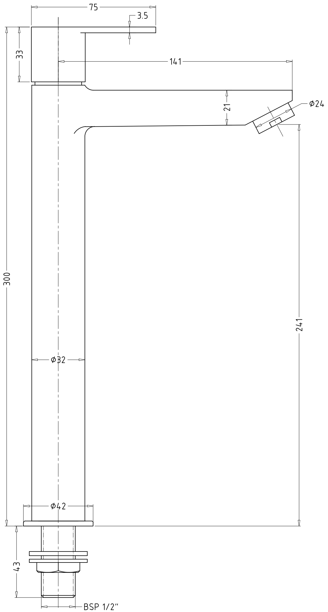
ASPIRO: 570002 PILLAR COCK TALL
